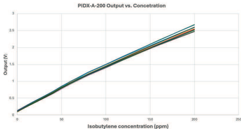
图1 PIDX-A-200 线性度 (0-200 ppm)
